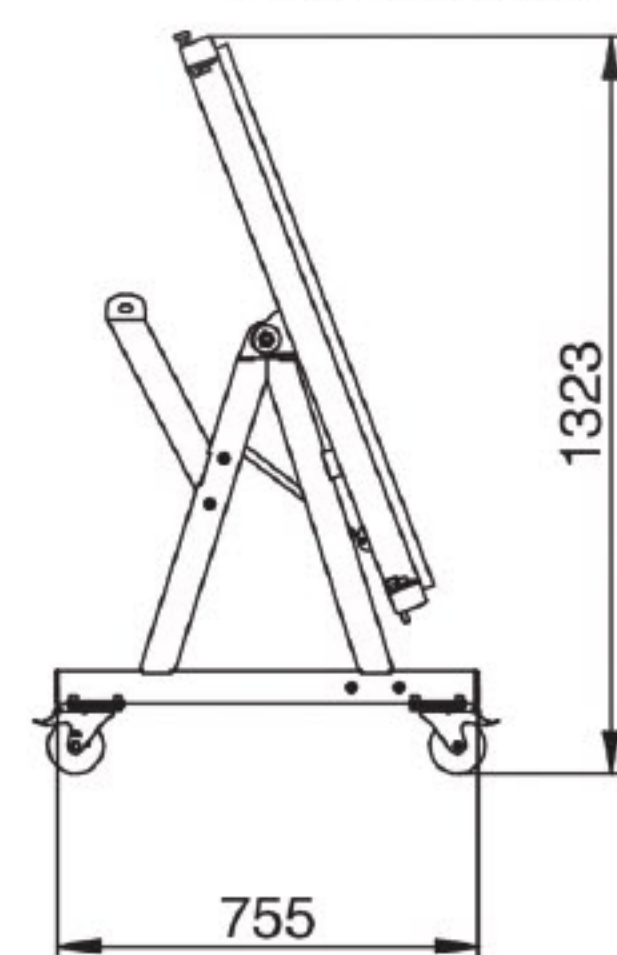
Stôl L2000 • 6x svorka SKP1100 • zásobník na uloženie svoriek • stolová doska
