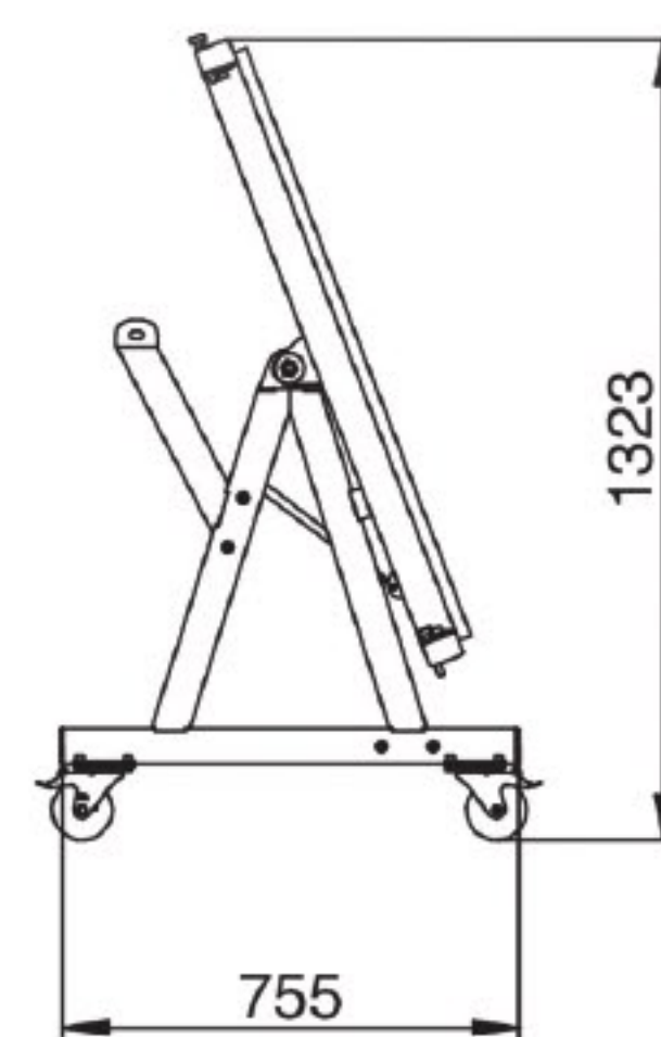
L2000-frame • 6x SKP1100 klem • tijdschrift • tafelblad
