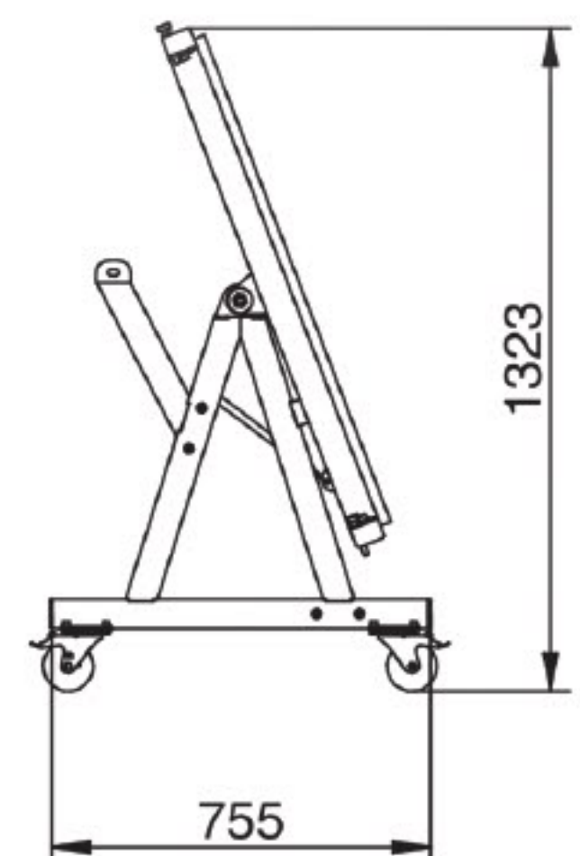
SKP - L2000 • 6 x SKP1100 • clamp storage • mdf top
