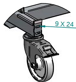
Szczegół A Otworowanie pod hak
