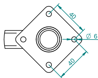
Szczegół A
