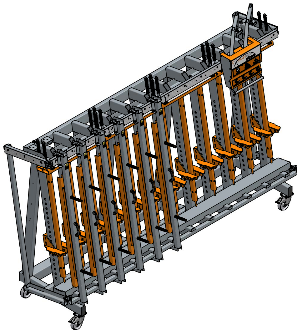
Prasa złożona
